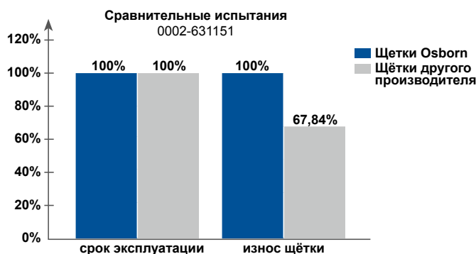
Результаты испытаний для чашечных щеток из жгутовой проволоки Osborn.
